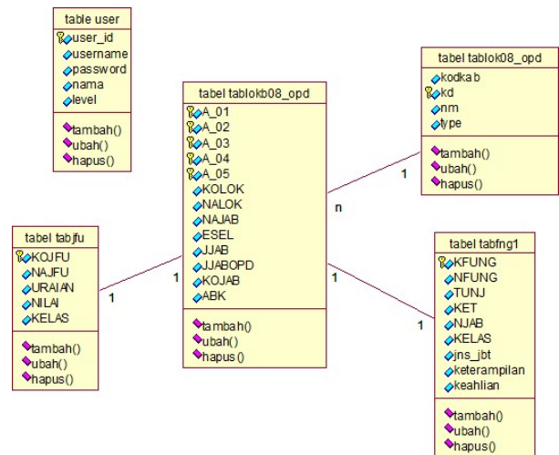
Gambar 2 Diagram Class Entitas Pada Sistem Pemetaan Jabatan
