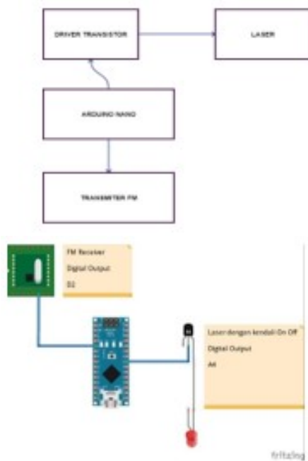
Gambar 5 Blok Diagram Pemancar
